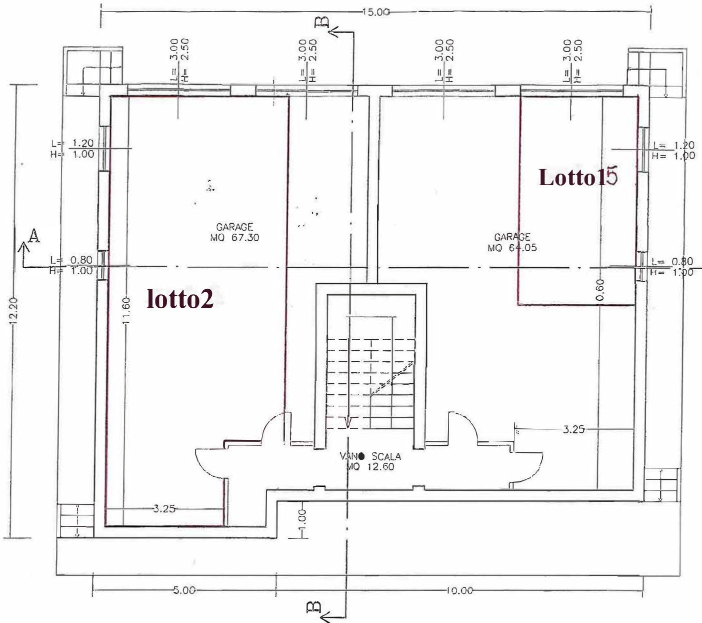
PIANTA PIANO INTERRATO
